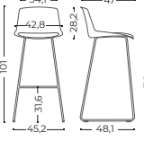
Cantilever stool Taburete Patín de acero
