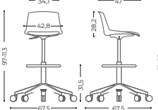
Draughtman chair Banqueta - Elevación gas
